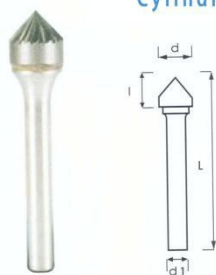
90° 圓錐形 (K 型) Cylindrical (Type K)
